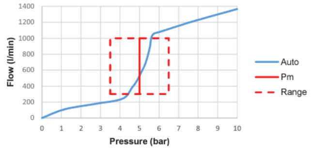
Handline FO6 PN 16
